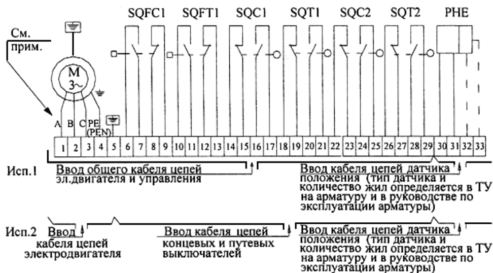
Рис.3. Электрическая схема соединения электропривода регулирующей арматуры
